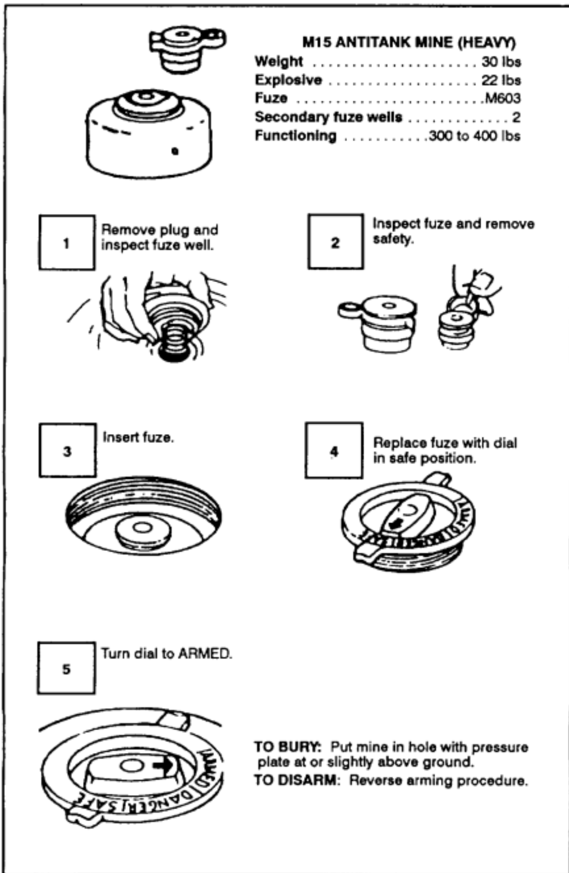
Figuer B-9. Antitank mines.
