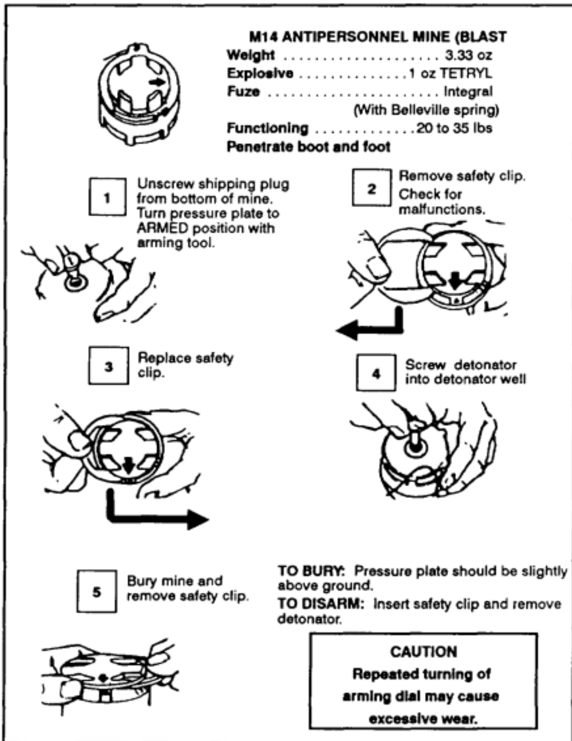
Figure B-8. Antipersonnel mines.
